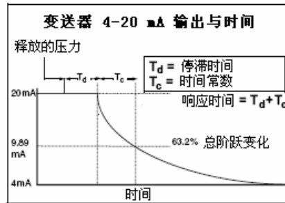
图 1 典型 HART 变送器响应时间
